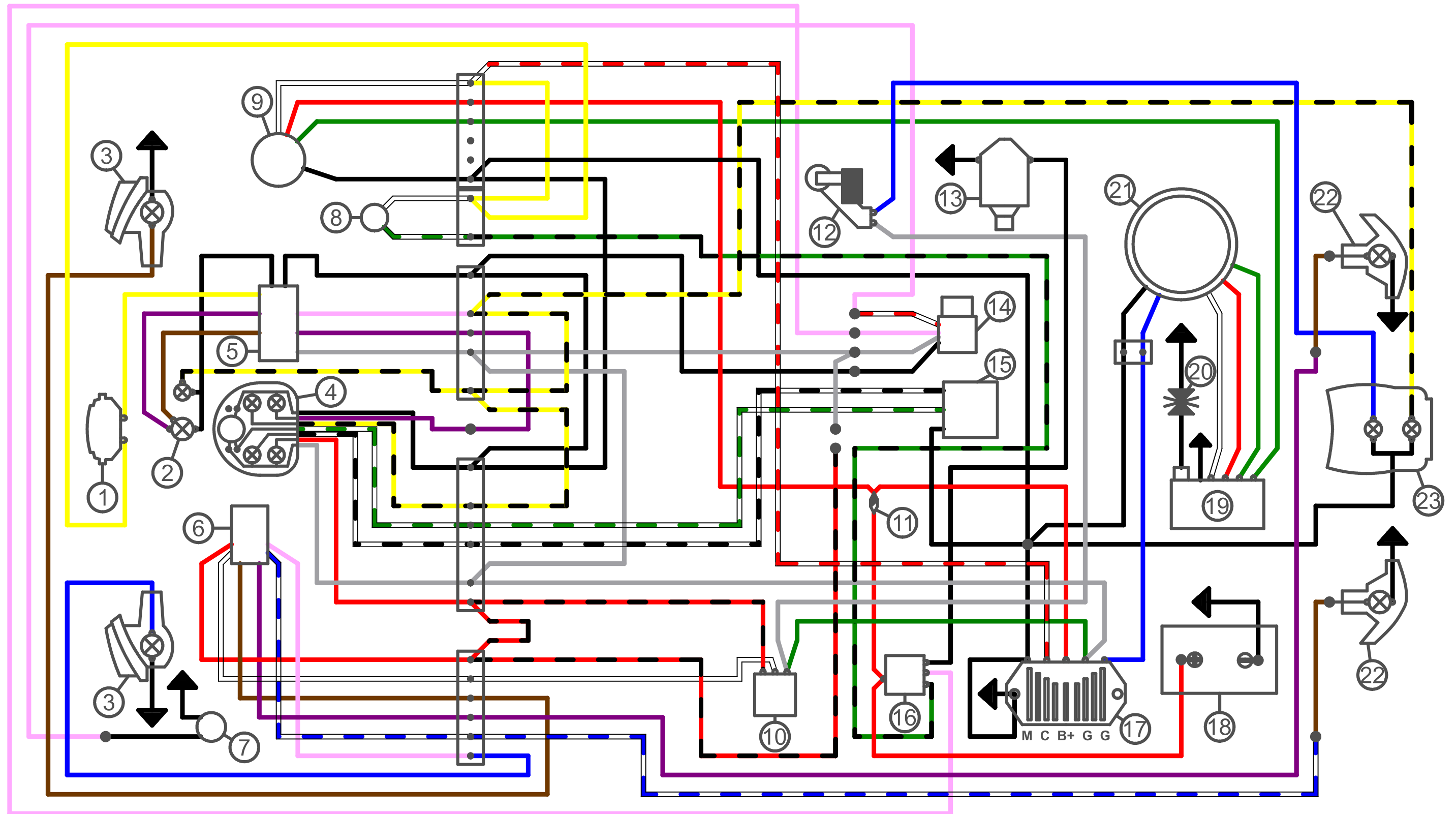
1 Hupe 2 Licht 3 Blinker 4 Tacho 5 Lichtschalter 6 Blinkerschalter 7 Kupplungsschalter 8 Anlasserknopf 9 Zündschloss 10 Blinkerrelais 11 Sicherung 12 Bremspedal 13 Anlasser 14 Starterkontrolle 15 Tanksensor 16 Starterrelais 17 Spannungsregler 18 Batterie 19 Zündeinheit 20 Zündkerze 21 Zündgrundplatte 22 Blinker 23 Rücklicht
